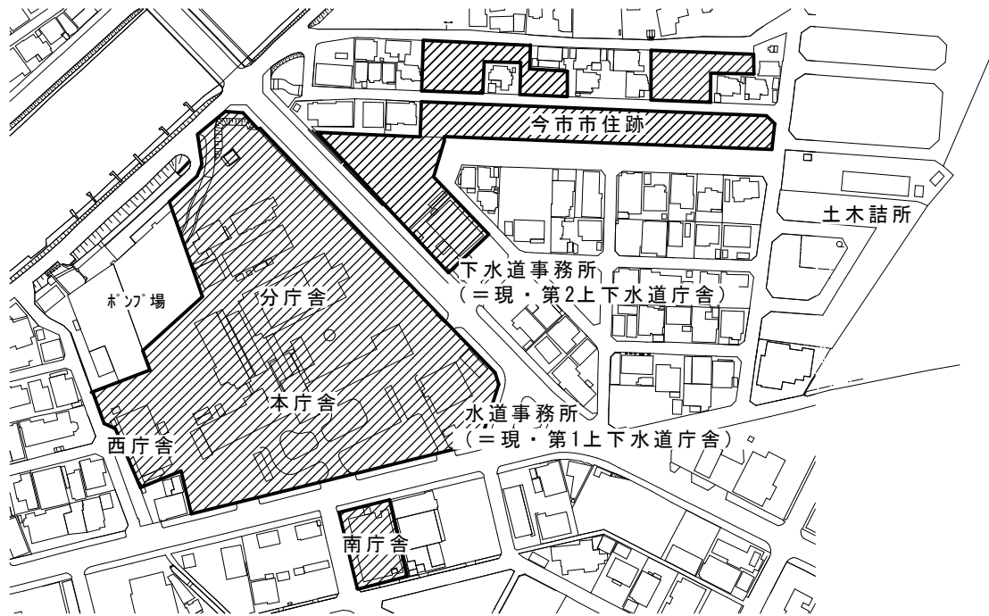
配置図 S=1/3,000
