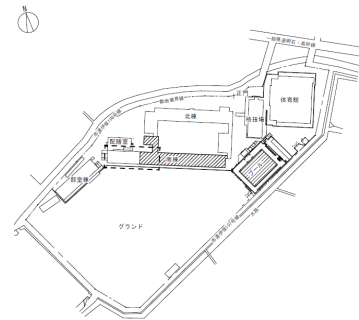
松陽中学校外壁及び防水改修工事計画図
