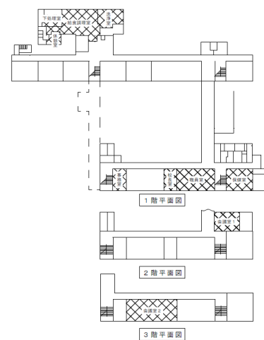
中筋小学校空調設備改修工事計画図
