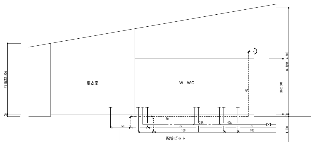
衛生設備系統図 S=N.S
