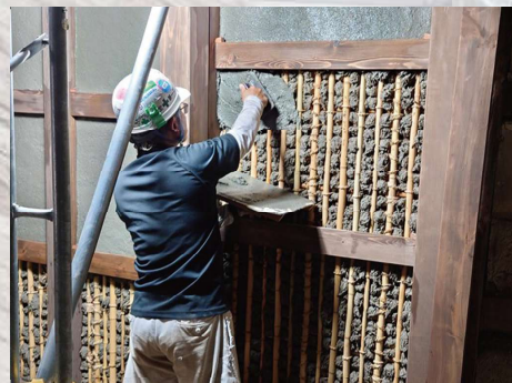
旧入江家住宅蔵 左官工事中
