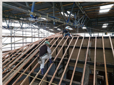
工楽松右衛門旧宅 屋根工事中
