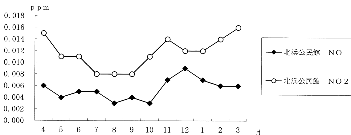
図 3-6 一酸化窒素及び二酸化窒素の月変化（平均値） 北浜公民館
