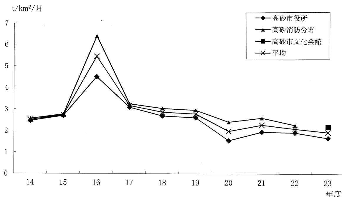
図 3-8 降下ばいじん量の年変化
