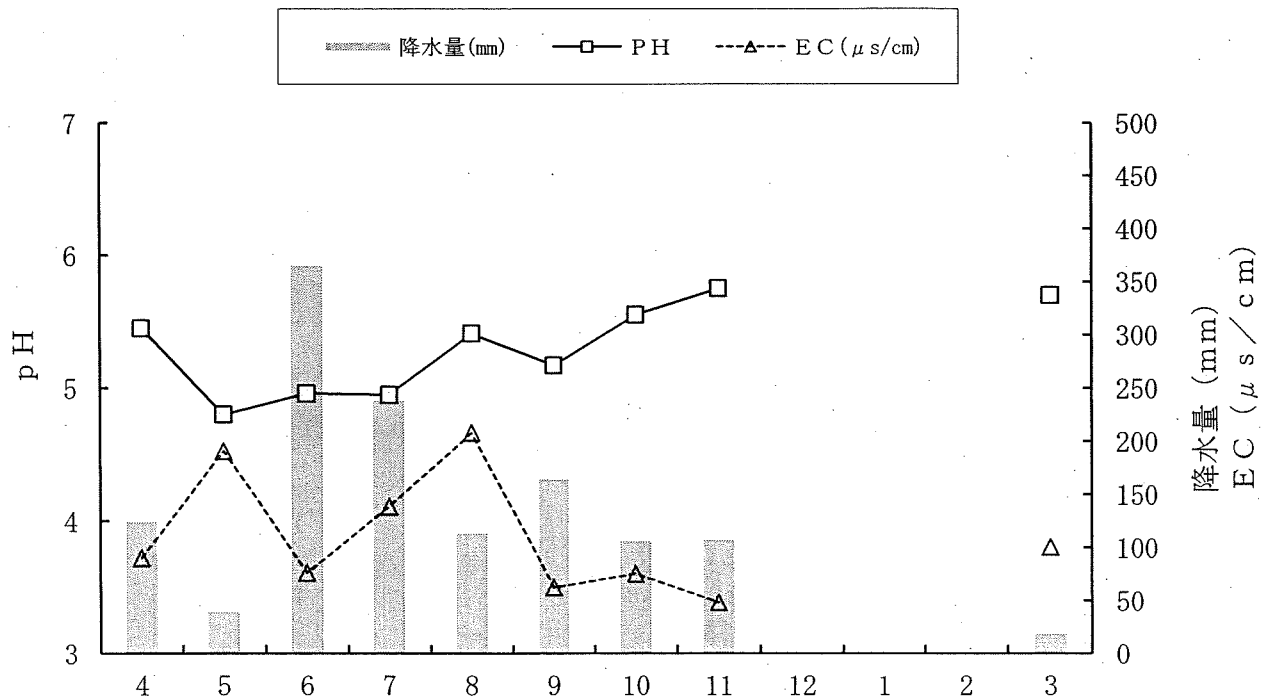
図 3-11 24年度酸性雨月変化
