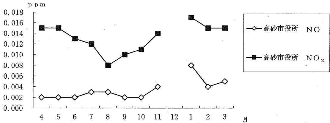
図 3-4 一酸化窒素及び二酸化窒素の月変化 (月平均値) 高砂市役所 ※12月は測定機故障により欠測
