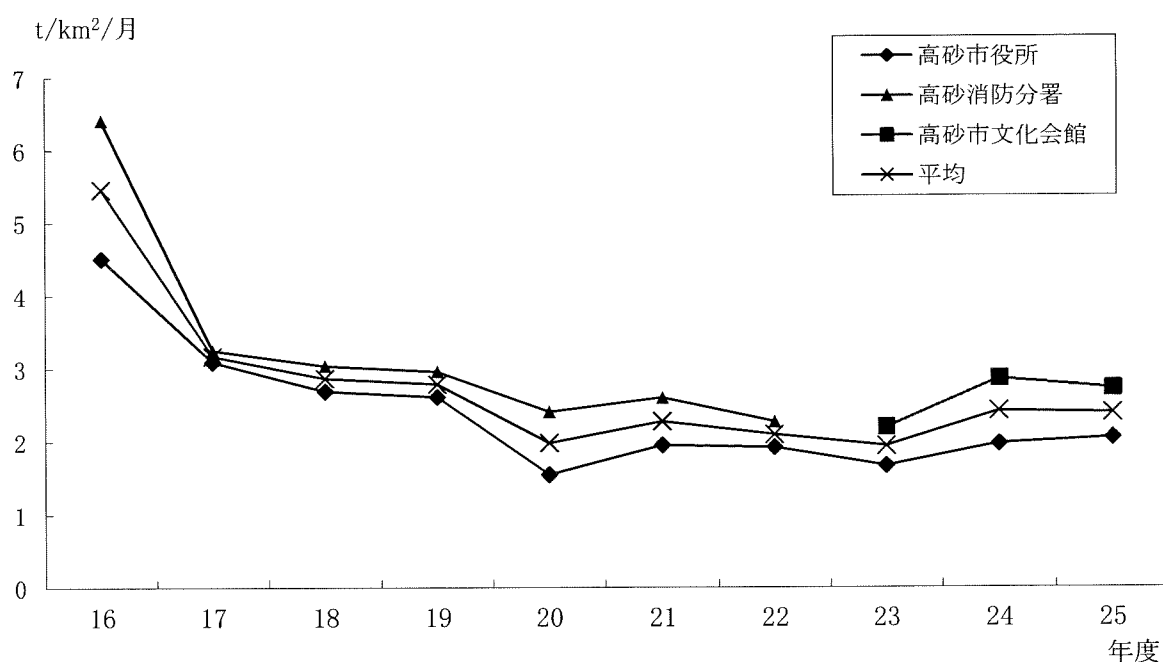
図 ３－８ 降下ばいじん量の年変化
