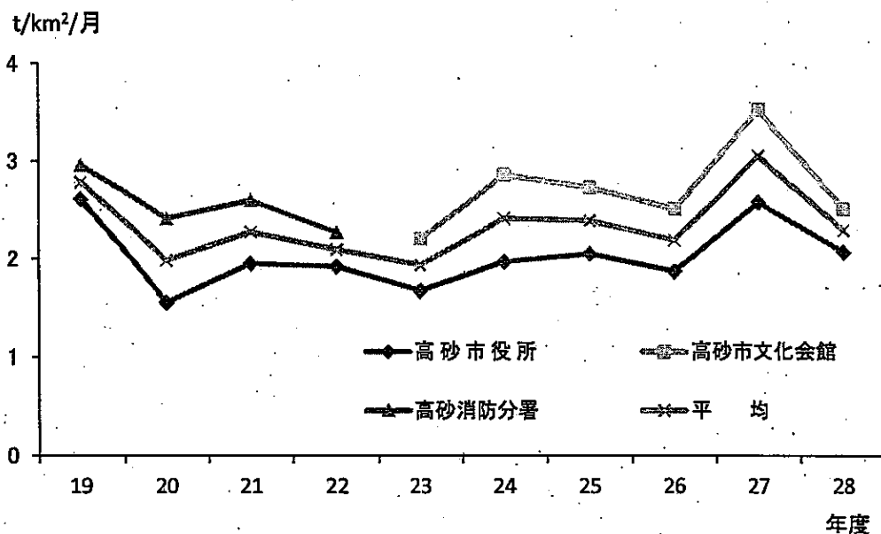
図 3-8 降下ばいじん量の年変化
