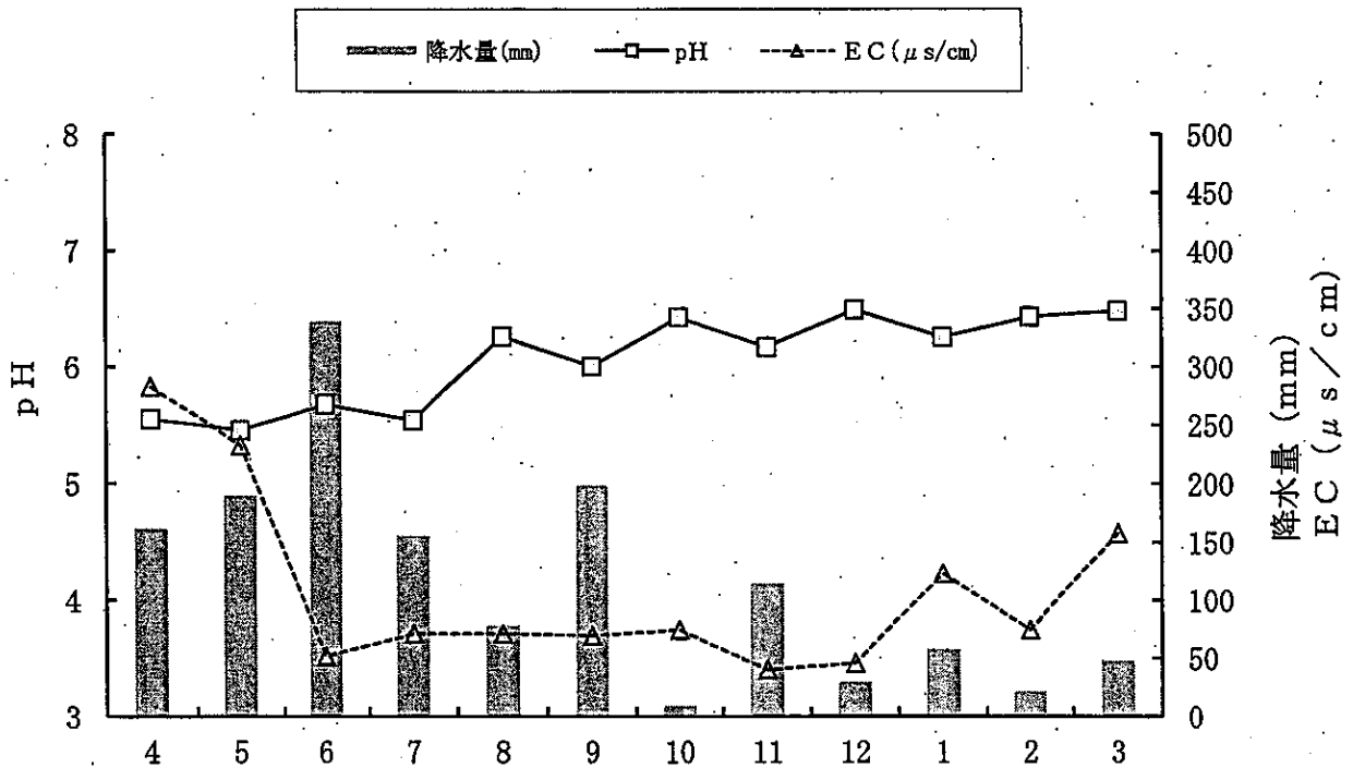
図 3-10 28年度酸性雨月変化
