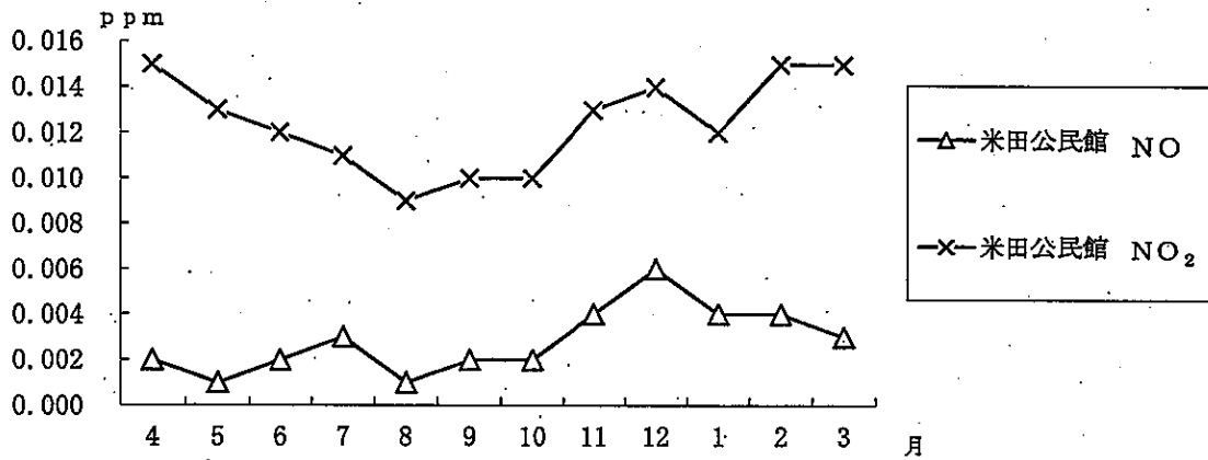
図 3-5 一酸化窒素及び二酸化窒素の月変化 (月平均値) 米田公民館
