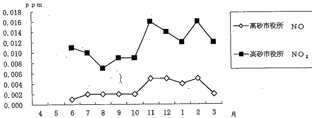
図 3-4 一酸化窒素及び二酸化窒素の月変化（月平均値） 高砂市役所 ※4月、5月は測定器異常のため欠測。
