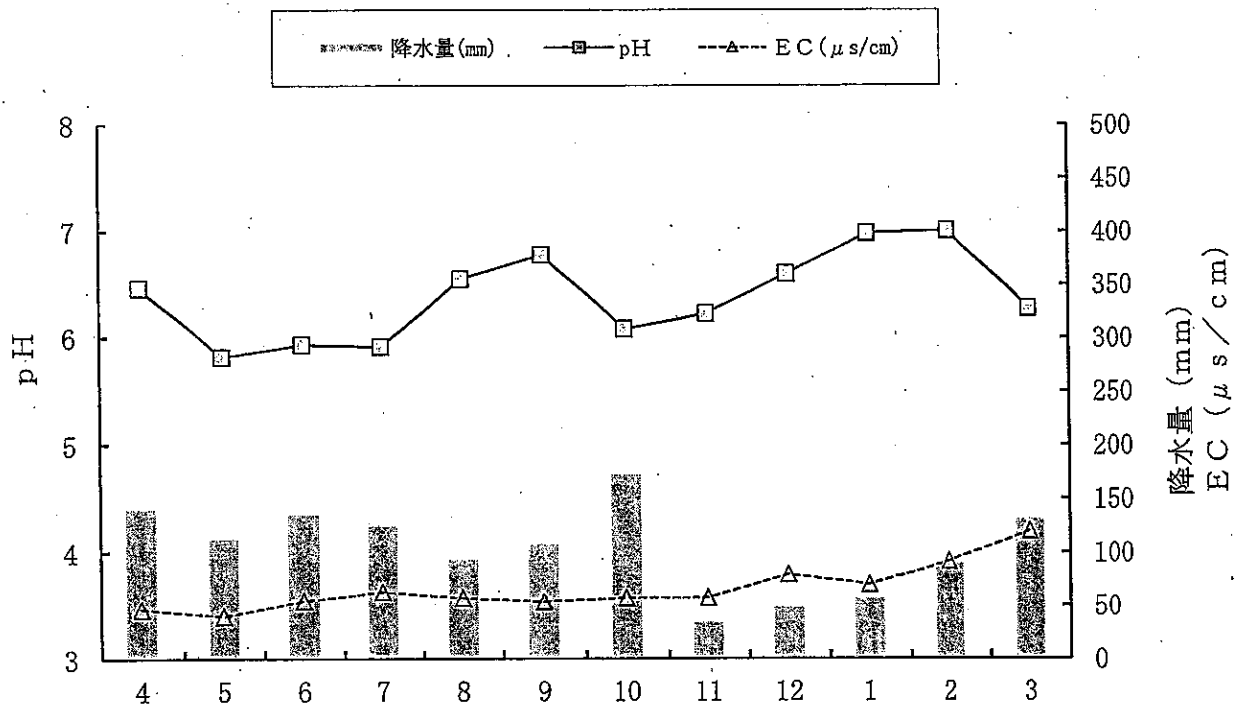
図 3-10 29年度酸性雨月変化
