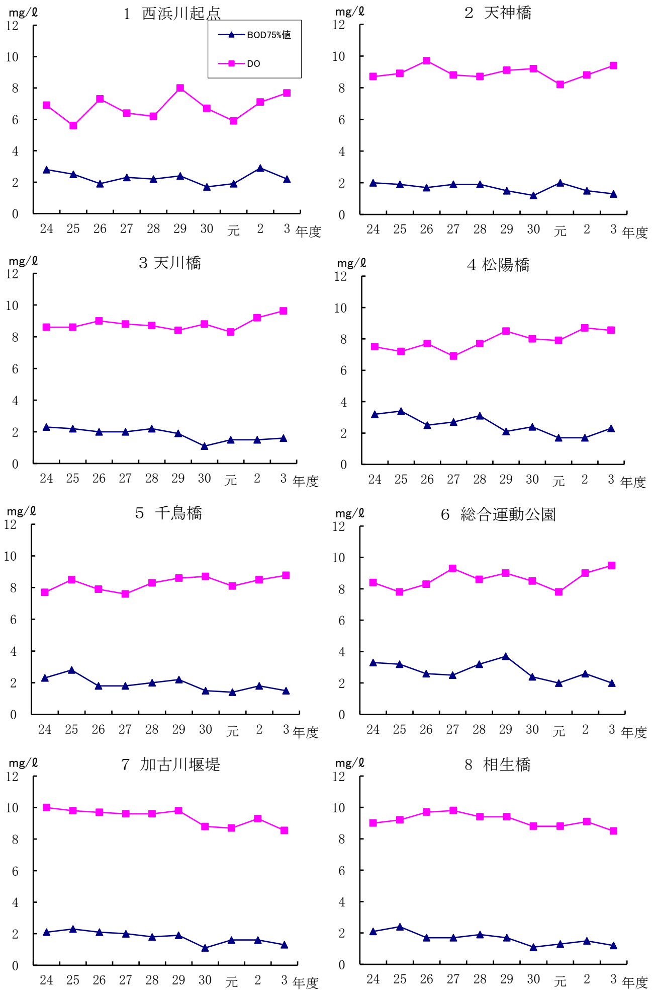
図4-3 調査地点別経年変化(BODは75%値・DOは年間平均値)
