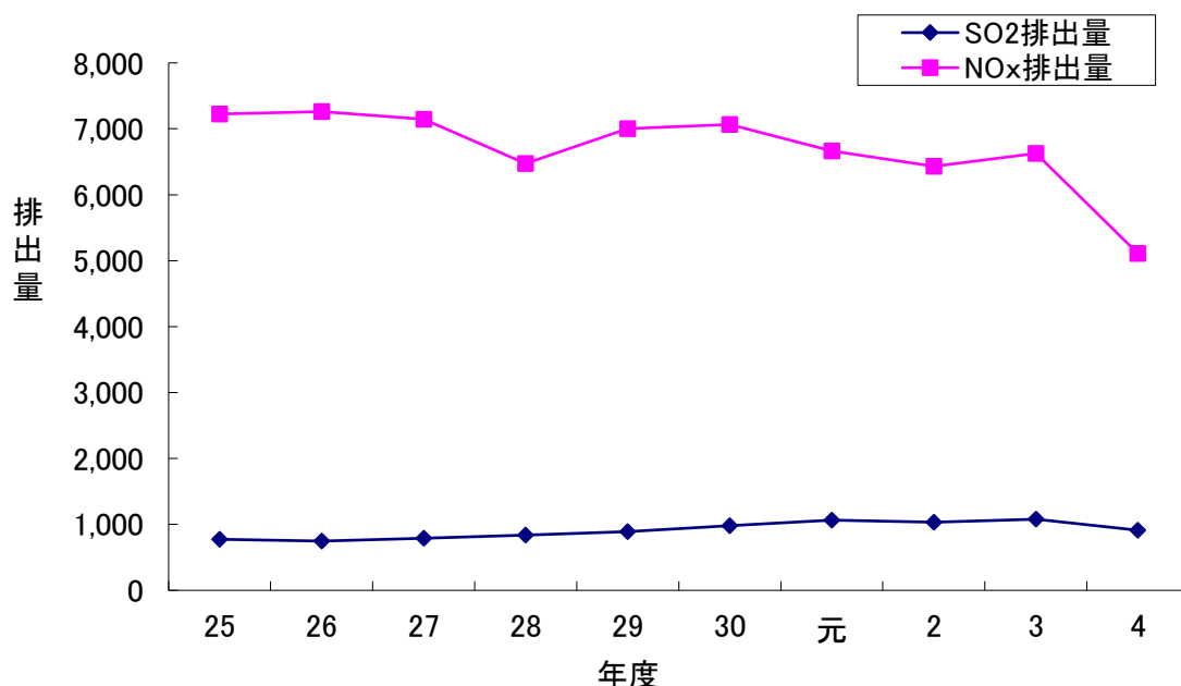
図 3-1 SO 2 及びNO x 排出量の経年変化
