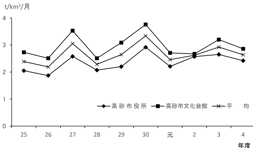
図 3-8 降下ばいじん量の年変化
